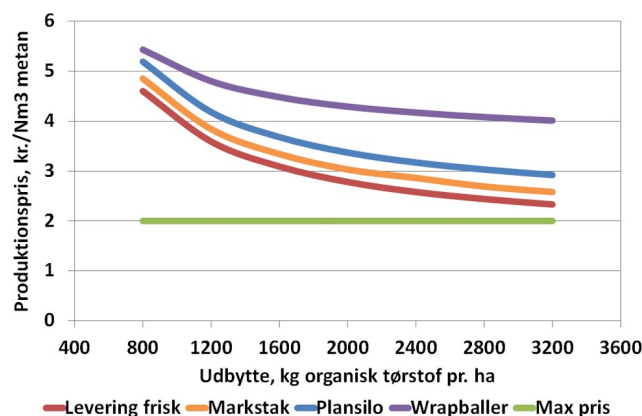
Figur 6. Produktionspris for ital. rajgræs som pligtig efterafgrøde til biogas an biogasanlæg afhængig af lagertype, kr. pr. Nm 3 metan. Beregnet ved et gaspotentiale på 300 Nm 3 pr. ton organisk tørstof pr. ha.
