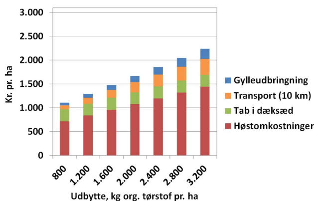
Figur 2. Produktionsomkostninger afhængig af udbytniveau for ital. rajgræs som pligtig efterafgrøde, der anvendes til produktion af biogas, kr. pr. ha. Biogasgylle returneres.
